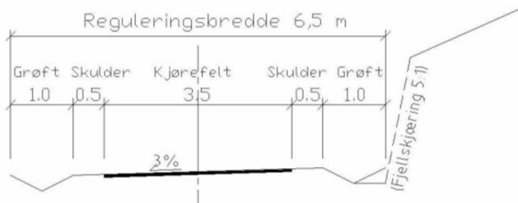
Fig. 8 snitt av planlagt adkomstvei.
