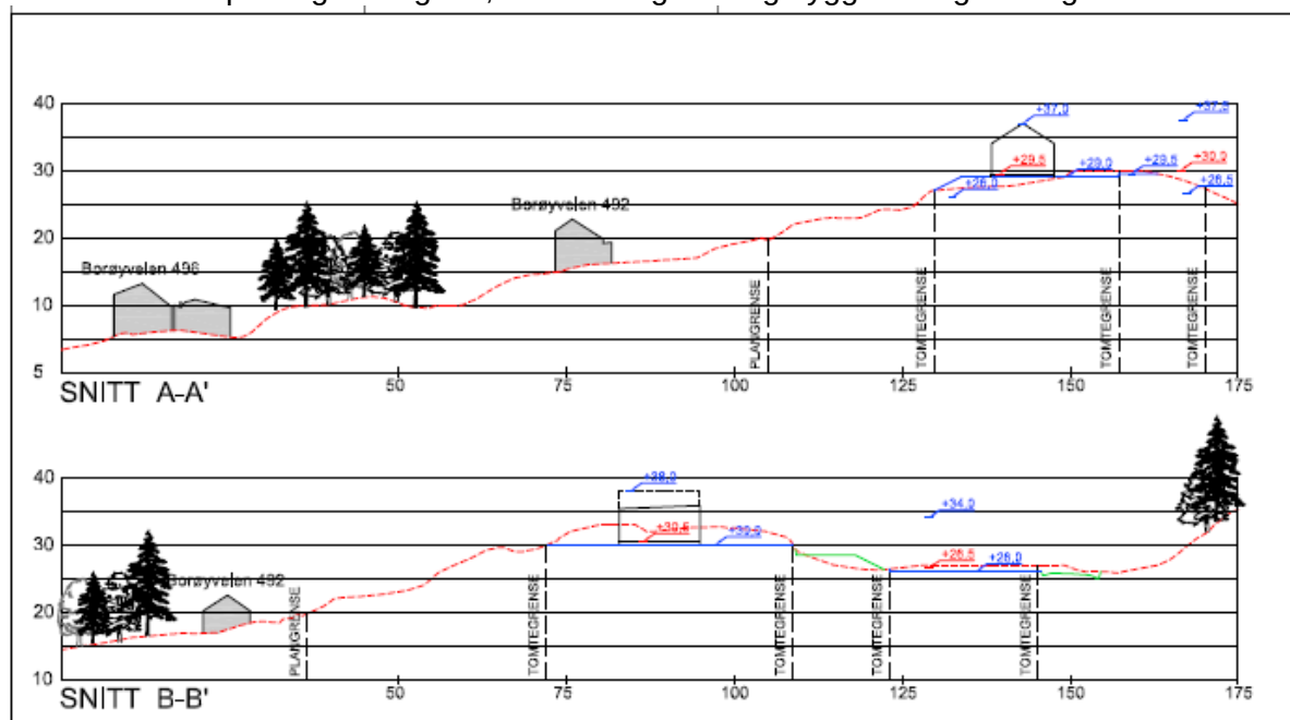
Figur 15 Snitt av planlagt utbygging.
