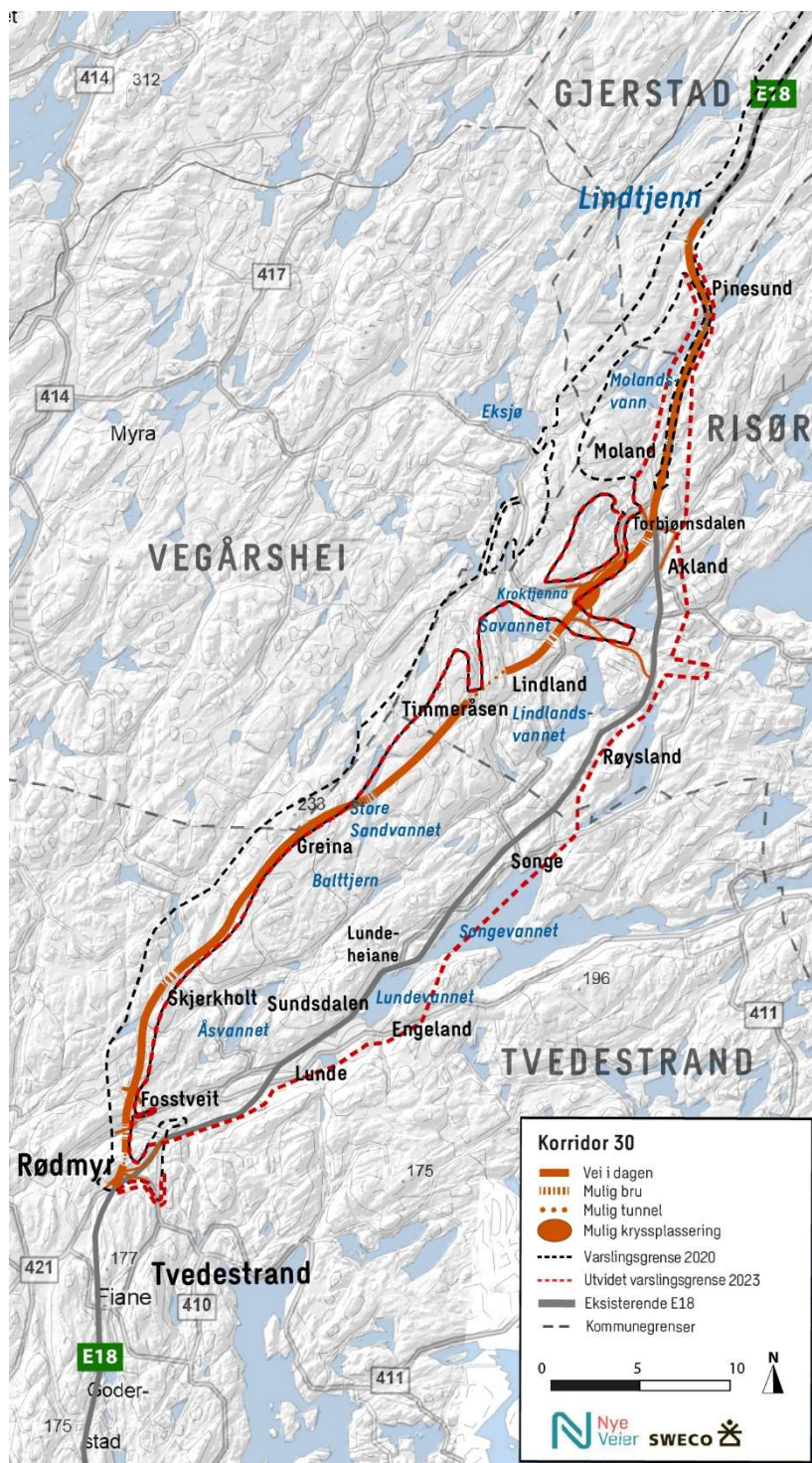
Figur 3-4: Figuren viser alternativ 30 med mulige kryssløsninger, broer, tunneler og lokalveinett.
