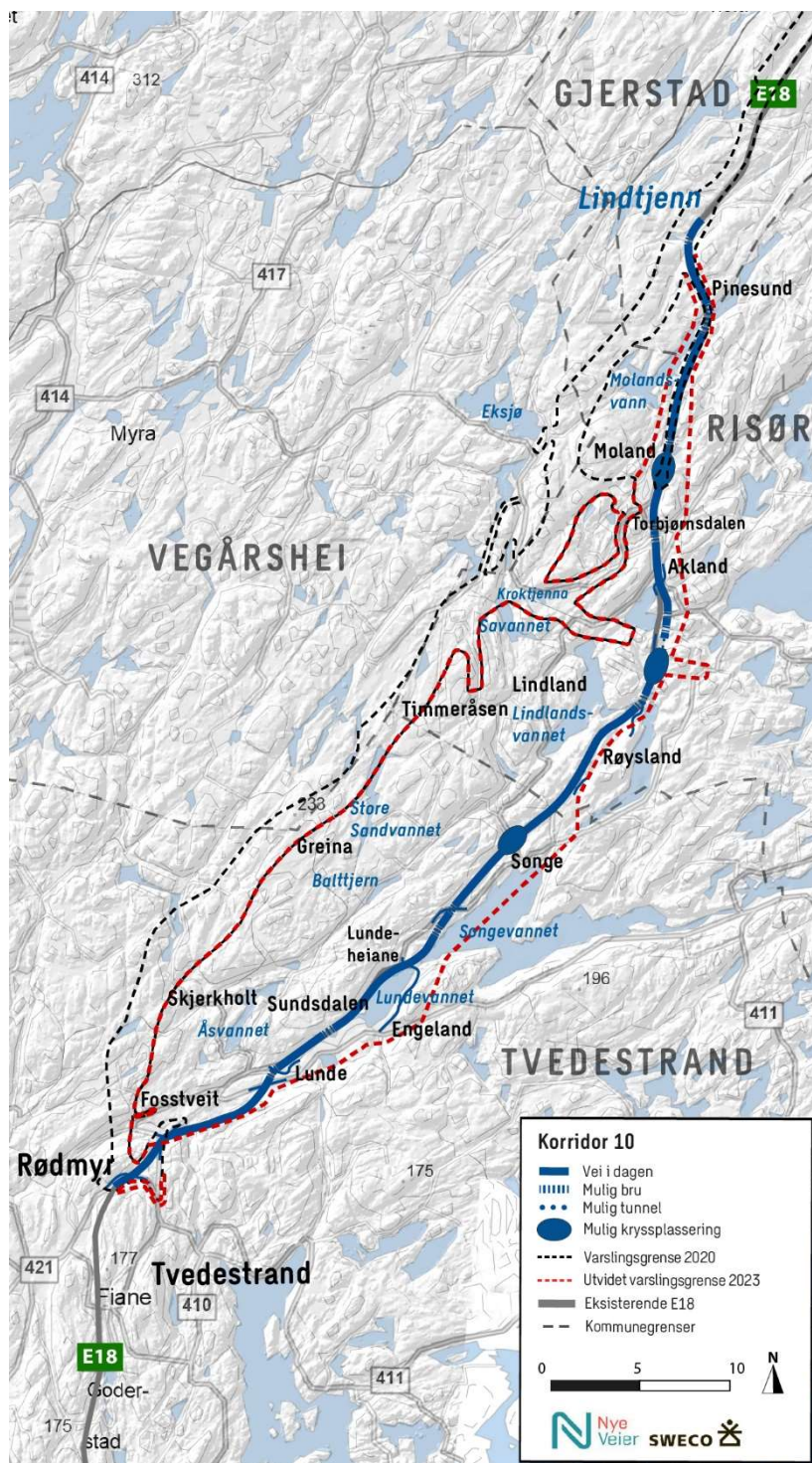
Figur 3-2: Figuren viser alternativ 10 - Gjenbruk av eksisterende E18 med mulige kryssløsninger, broer, tunneler og lokalveinett.
