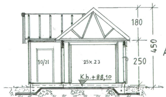
SNITT A
