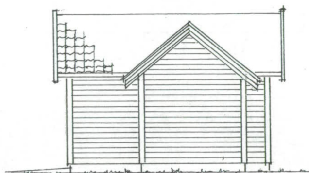
Fasade øst-syd-øst
